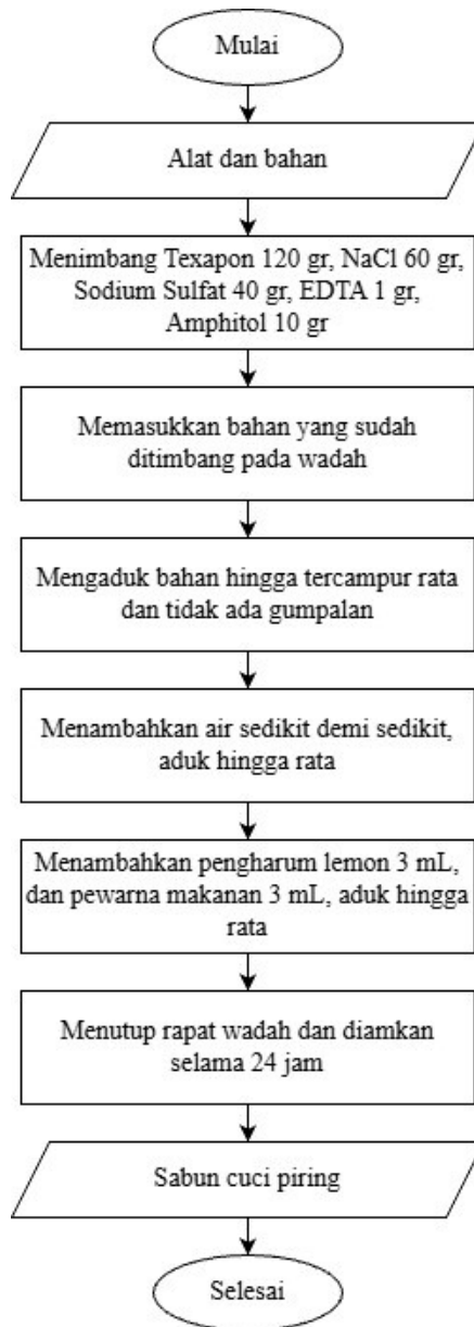
Gambar 1. Flowchart Pembuatan Sabun Cuci Piring
